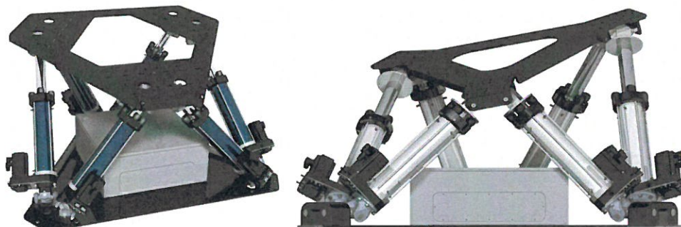
Obraz 3-1: Przykład platformy ruchomej z pomiarem zakresu ruchu symulatora
